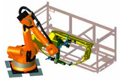
Roboterführung
